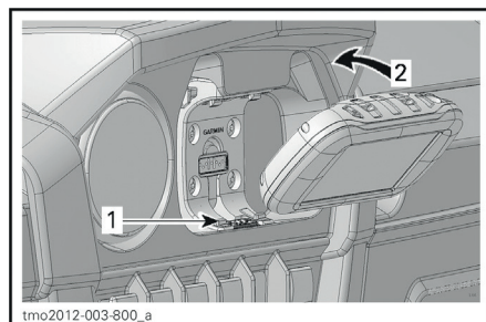
1. Нижняя лапка держателя
