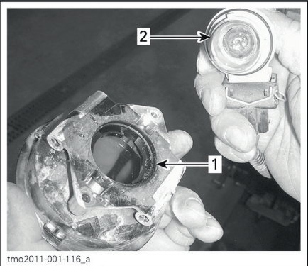
1. Задний фонарь
