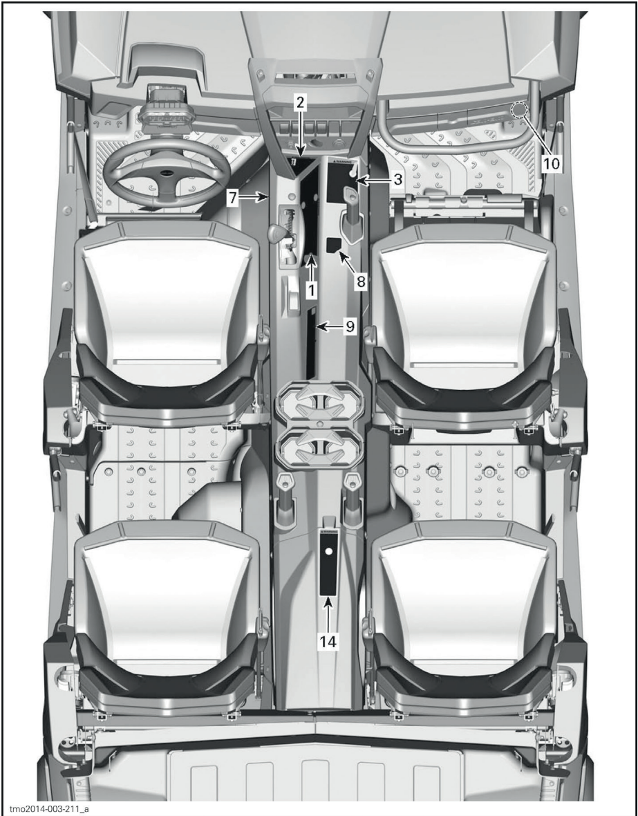
ТИПОВОЙ ВАРИАНТ – МОДЕЛИ DPS И XT
