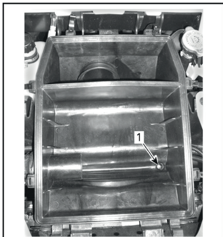
1. Сливное отверстие
