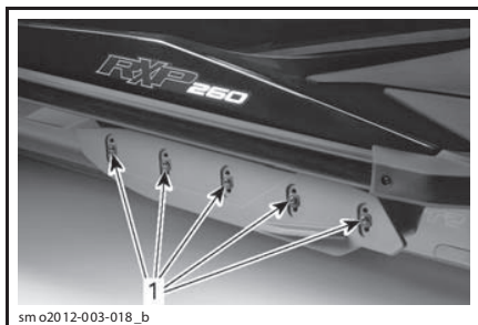
1. Самоостопоряющиеся винты
