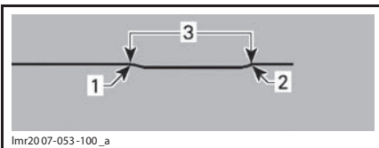
1. метка FULL (максимальный уровень масла) 2. метка ADD (требуется долив) 3. Рабочий диапазон
